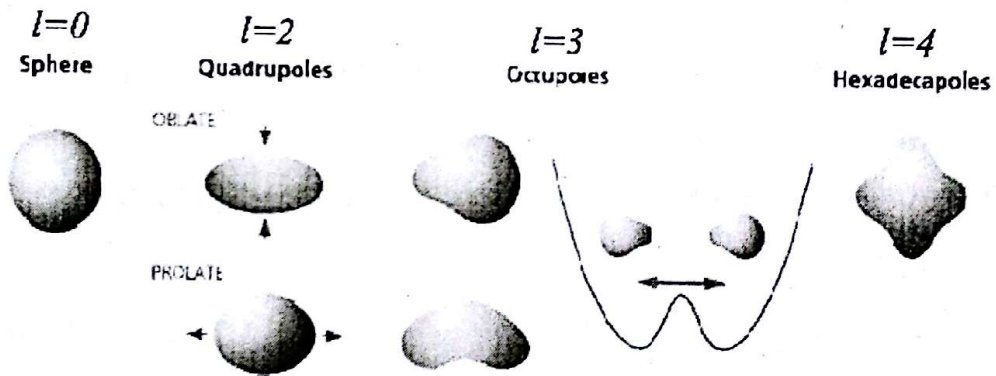
图1 l = 0, 2, 3, 4 时原子核的 2^l 极形变的形状示意图
